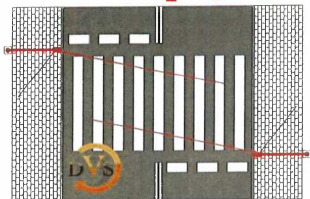
wysokość oprawy: 5m odległość oprawy od przejścia: 0m lampa ze średnim zasięgiem
