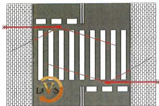
wysokość oprawy: 5m odległość oprawy od przejścia: 0m lampa z długim zasięgiem do środka pasa jezdni
