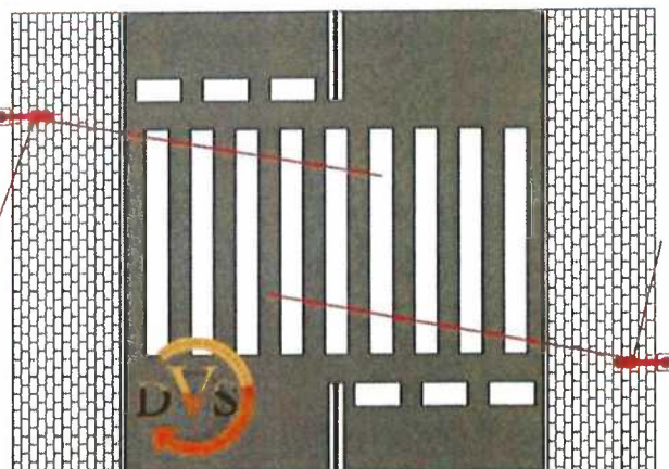
wysokość oprawy: 5m odległość oprawy od przejścia: 0m lampa z krótkim zasięgiem
