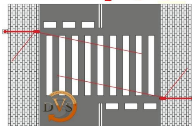
wysokość oprawy: 5m odległość oprawy od przejścia: 0m lampa ze średnim zasięgiem
